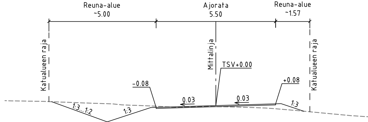
TYYPPIPOIKKILEIKKAUS AIKKALANTIE (PL 180) 1:100
